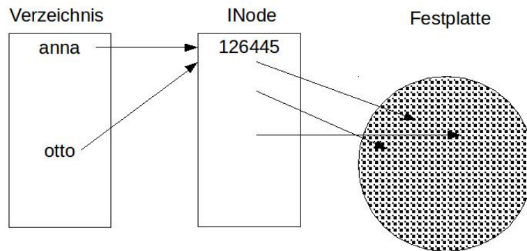
Abbildung 3: Inodes
